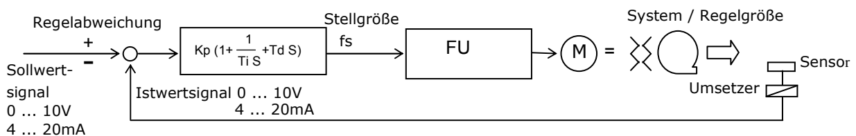
Kp:Proportionalbeiwert, Ti:Nachstellzeit, Td:Differenzierzeit, s:Frequenzvariable
