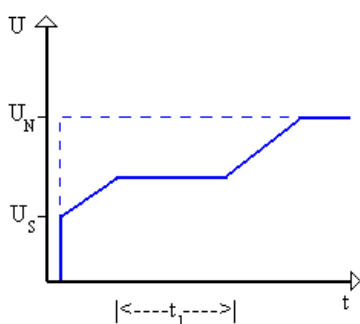
2-8 Klemmenspannung des Motors mit Strombegrenzung
