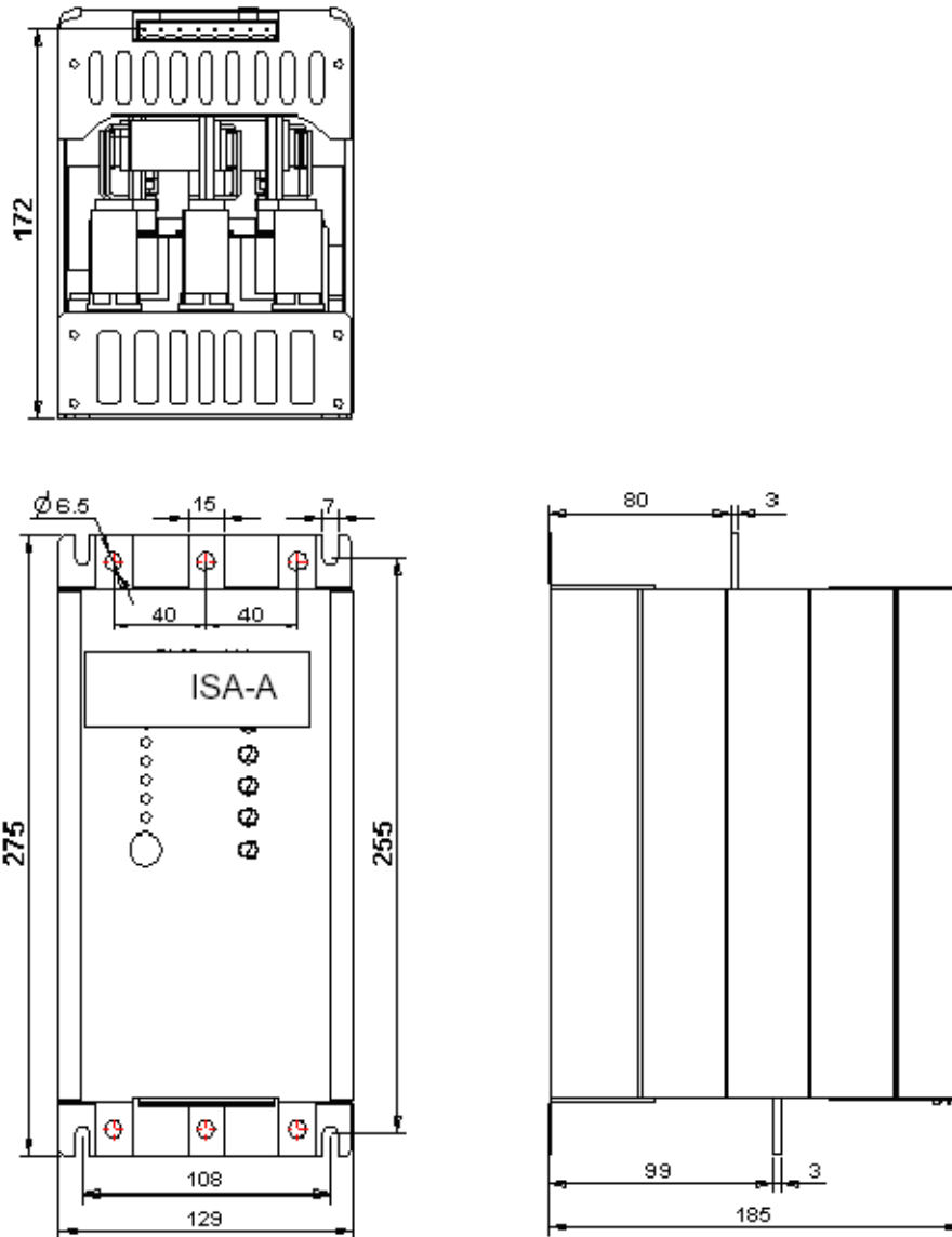
10-2 Dimensionszeichnung Gehäuse A2
