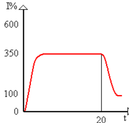
6-3 Strombegrenzung
