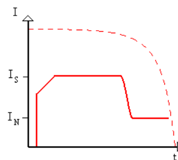
2-9 Stromverlauf mit Strombegrenzung
