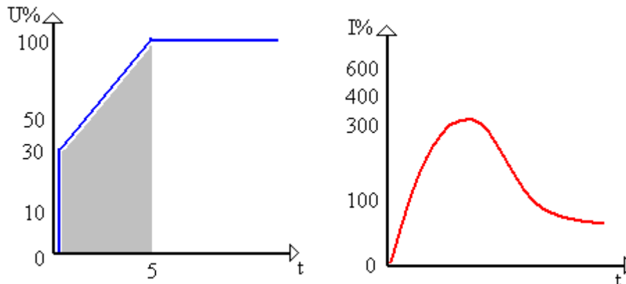
6-6 Beispiele von Startkurven 1
