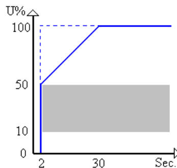
6-2 Startmoment
