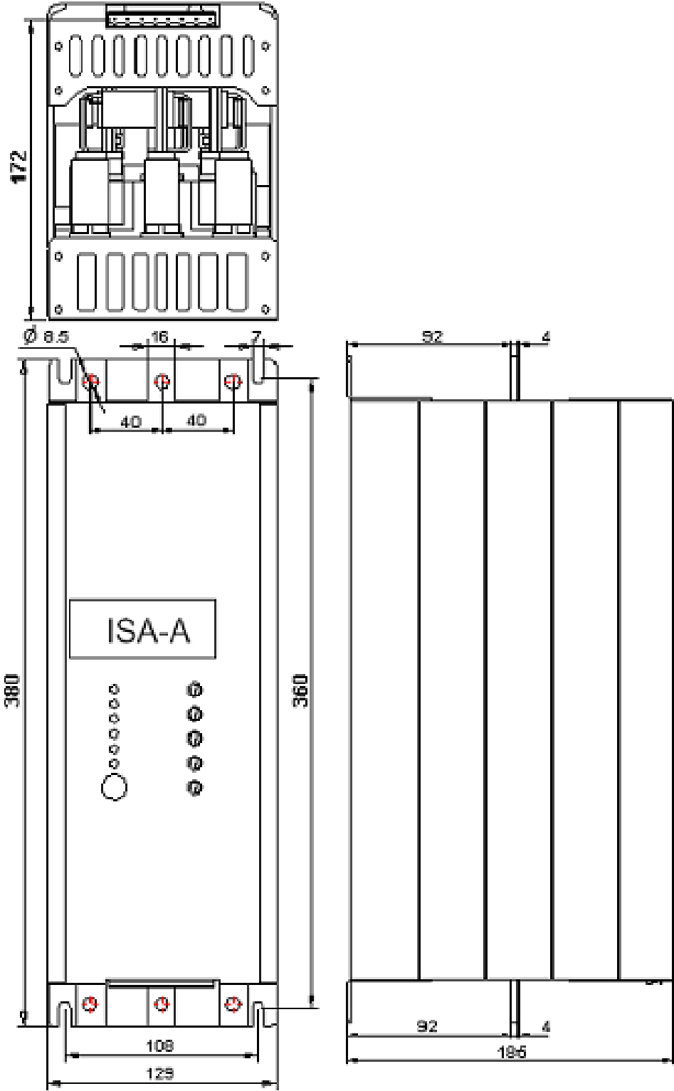
10-3 Dimensionszeichnung Gehäuse A3
