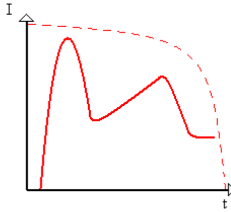
2-11 Stromverlauf Boost-Start
